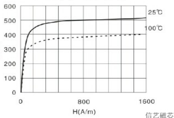
B-H 磁化特性曲线 B-H Loop (at 25°C 100°C)
